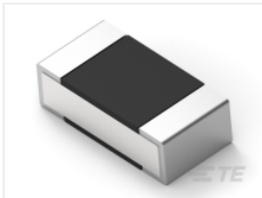
TE 产品编号3-2176305-6 RP 1E 0.1W 249R 0.1% 25PPM 5K RL
