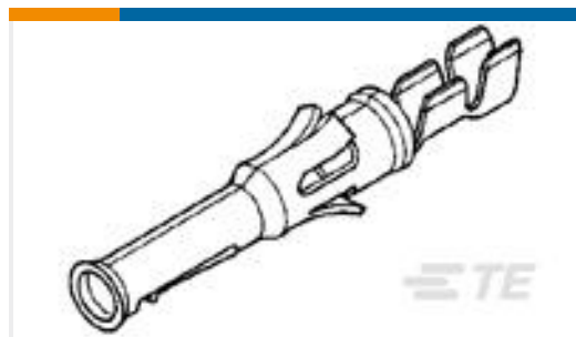
TE 产品编号66594-1 TYPE VI SKT CONT,MULTIMATE
