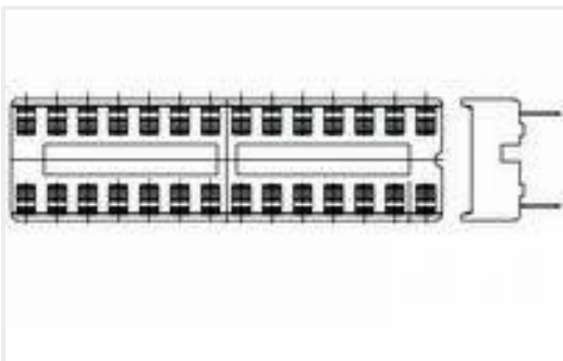
TE 产品编号1-2199298-3 14P,DIP SKT,300 CL,LDR,PB FREE
