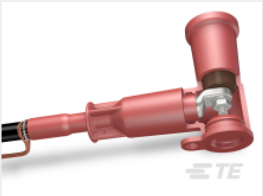
TE 产品编号 CM2361-011 RICS-3133
