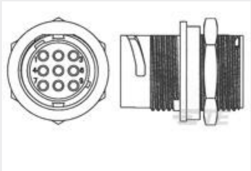
TE 产品编号1445823-3 REC,11-6,FLNG MT,LG INS,STD KE
