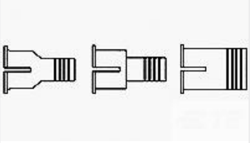
TE 产品编号6-745129-9 SHILDING FERRULE,PLTD,BULK PKG
