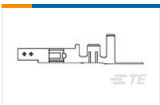
TE 产品编号794956-1 VAL-U-LOK SKT BR SN 22-18AWG BR
