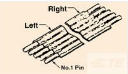
TE 产品编号5-1437141-1 FSN-22.5A-4="FLXSTRP NMX .100
