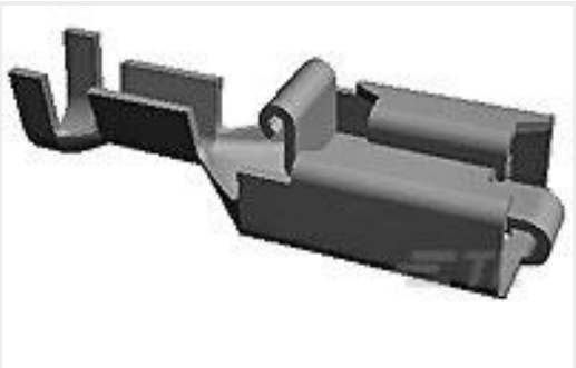
TE 产品编号880645-6 PL REC 1.0-2.5MM2 0.40 X 52.32 PTPBR
