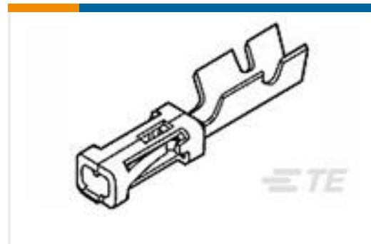
TE 产品编号6-87756-2 MOD IV RECP PLTD 15 DPLX LF
