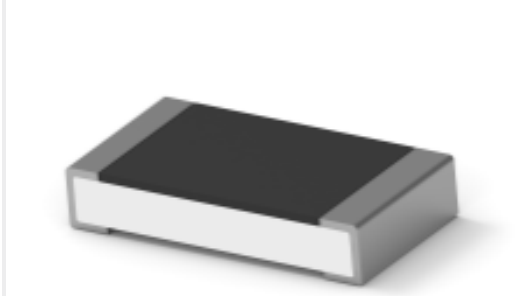
TE 产品编号1-2176389-2 RQ 1206 140R 0.1% 10PPM 5K RL
