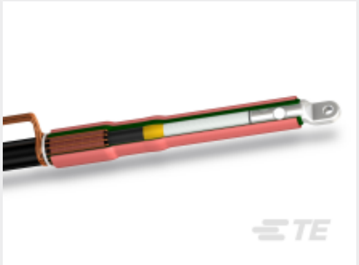
TE 产品编号CF6351-005 IXSU-F3131-ML-4-13
