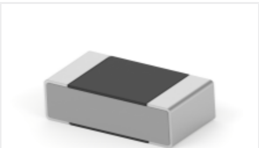
TE 产品编号8-1879140-4 RN 0603 137K 0.1% 10PPM 5K RL
