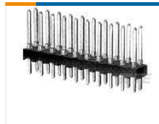
TE 产品编号87227-3 06 MODII HDR DRST UNSHRD .100
