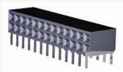
TE 产品编号 2-535512-0 26 MODII HORZ DR CE EESS .100
