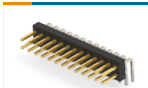
TE 产品编号 6-103326-3 26 MODII HDR DRRA B/A .100CL
