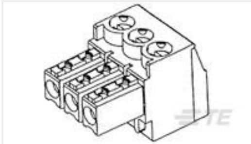
TE 产品编号284507-8 8 POS TERMI-BLOK PLUG STAC 3,8
