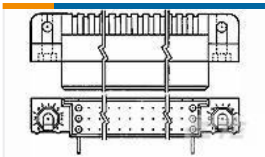
TE 产品编号 533268-1 HDI RECP ASSY 3 ROW 75 POS
