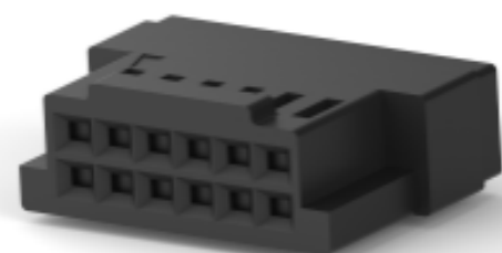
TE 产品编号 CAT-F439-R2435254 2.54mm FFC 连接器母端外壳
