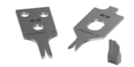
TE 产品编号 7-2151980-7 OCEAN_2.0_SPARE_PART_KIT-055F062O
