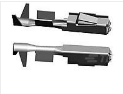
TE 产品编号5-928999-6 MQS0,63 Ag rec LL unseal. >0,2-0,35
