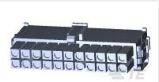
TE 产品编号794212-1 22P MINI UMN L2 PLUG HSG UL94V0
