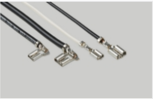
快速断开(213)
