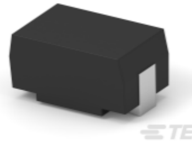
TE 产品编号5-1879234-2 SMD 功率电阻器：7 瓦特，200-2M 欧姆
