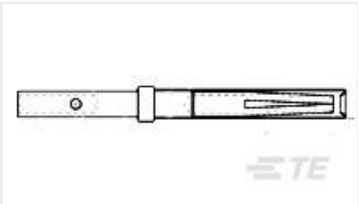
TE 产品编号208264-2 SKT CONTACT SZ 22
