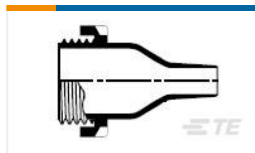
TE 产品编号878118-000 207W245-3/42-0
