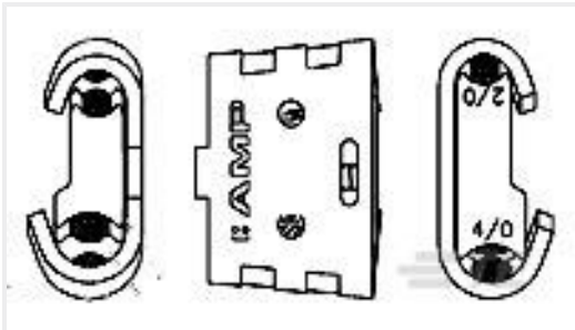
TE 产品编号83631-7 MINIWEDGE,200AMP,2/0-#2
