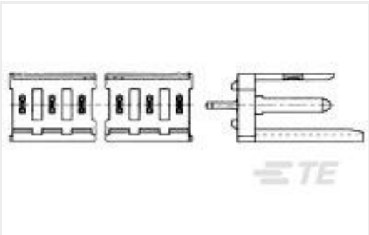
TE 产品编号 280615-1 02P MOD 1 ASSY.
