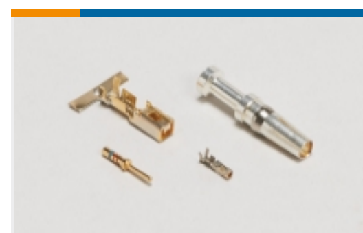
连接器端子(64)
