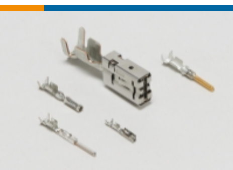
汽车端子(137)
