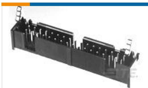
TE 产品编号2-1761608-6 IDC LOW PRO HDR 16P VERT SHT L
