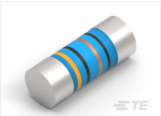
TE 产品编号5-2176315-1 MELF SMA_A 1K2 1% 50PPM 0204 0.4 W
