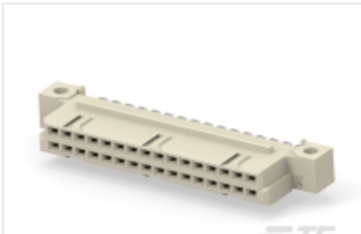
TE 产品编号294722-E STVQ/2 32 FI AB VV 7-03 TL ** 247 E 172
