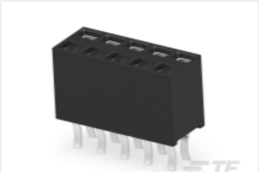
TE 产品编号 215308-5 2X 5P HV100 REC CON. TE, 7.0MM, TIN
