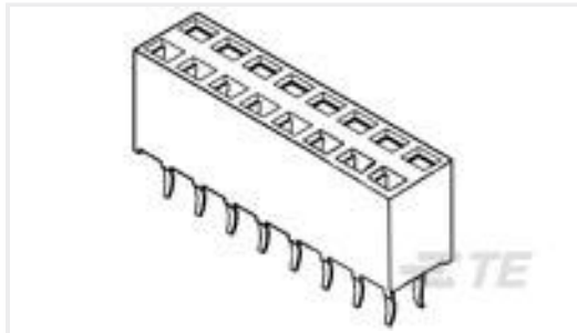
TE 产品编号 215310-5 2X5P HV100 REC CON. TE, 8.5MM, TIN
