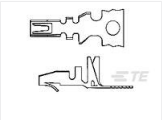
TE 产品编号3-794122-1 MINI AMPIN 2000,26-22AWG,PHBRZ
