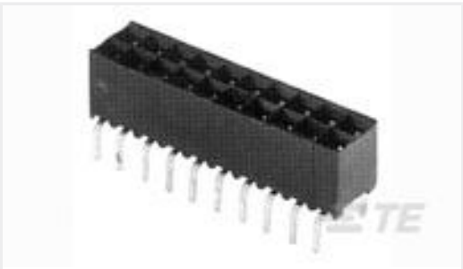
TE 产品编号 829264-5 2X 5P HV100 REC CON.B/TE, 6.2,NO KINK
