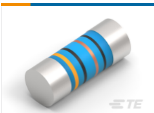
TE 产品编号2176314-9 MELF SMA_A 470R 0.1% 15PPM 0102 0.3W
