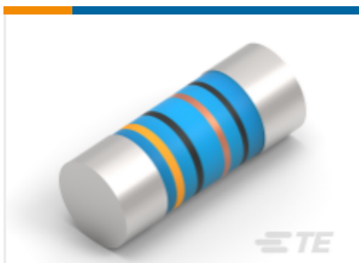
TE 产品编号2-2176314-2 MELF SMA_A 5K6 0.1% 15PPM 0102 0.3W
