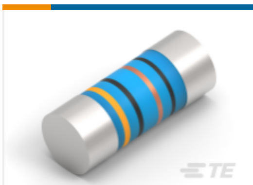
TE 产品编号3-2176314-0 MELF SMA_A 27K 0.1% 15PPM 0102 0.3W
