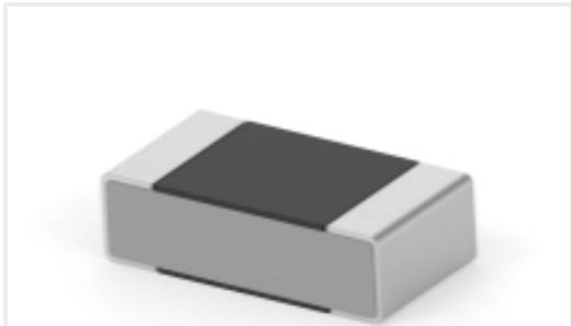
TE 产品编号1-1879207-1 RN 0603 255K 0.1% 10PPM 5K RL
