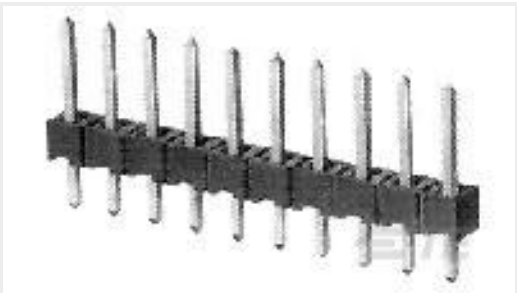
TE 产品编号354081-E SMCQ 40 F AB VV 7-03 CL * 0007 137 E002
