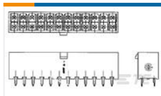
TE 产品编号1586037-4 4P VERT HDR VAL-U-LOK V2
