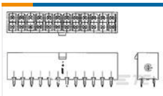
TE 产品编号1586038-4 4P VRT HDR VAL-U-LOK V0
