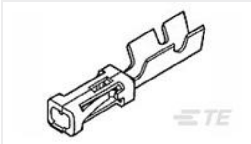
TE 产品编号166310-2 MOD-5 REC.CONTACT
