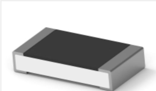
TE 产品编号6-2176391-5 RQ 1206 57K6 0.1% 10PPM 5K RL
