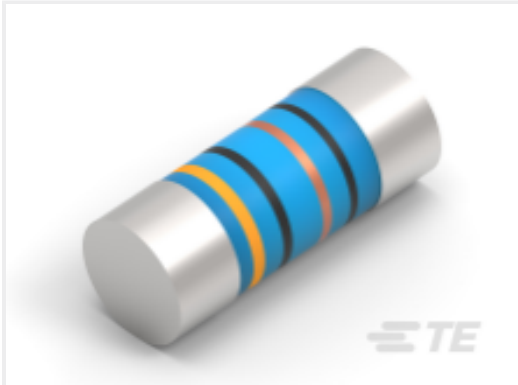
TE 产品编号3-2176316-4 MELF SMA_A 56K 0.1% 15PPM 0207 1W
