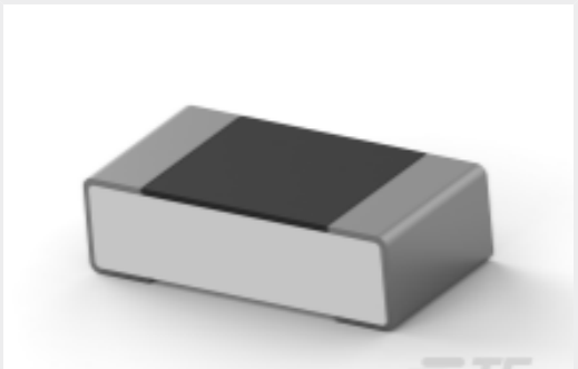
TE 产品编号1-2176369-0 RQ 0603 49R9 0.1% 10PPM 5K RL
