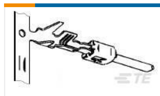
TE 产品编号2-2141598-2 TAB 2.8x0.8 CONTACT CF SRC Ag
