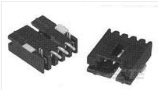
TE 产品编号5-147278-7 08 MTE HDR SRRA SFMNT .100CL
