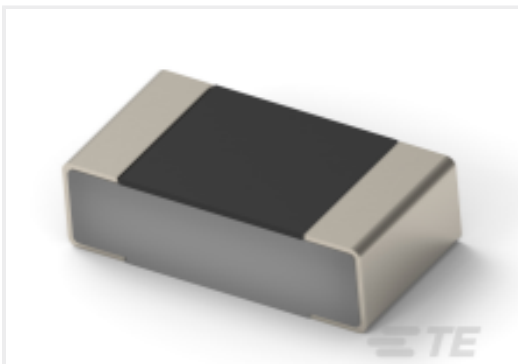
TE 产品编号5-1879808-1 RP 1J 0.1W 392K 0.1% 15PPM 1K RL
