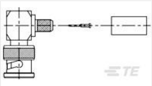
TE 产品编号1-1478075-0 BNC R/A Plg Hex 50Ohm Silver Pltd RG58C/
