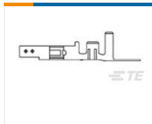
TE 产品编号794956-1 VAL-U-LOK SKT BR SN 22-18AWG
