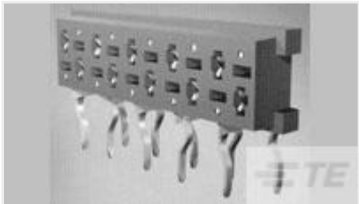
TE 产品编号 8-100400-0 MICRO-MATCH FSID NP
