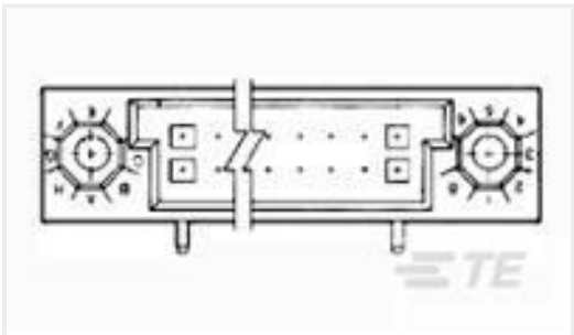
TE 产品编号1-532825-4 HDI RECP ASSY 2 ROW 150 POS
