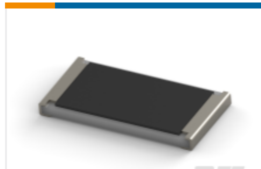
TE 产品编号7-2176070-5 SMD 功率电阻器：2 瓦特，3521 系列
